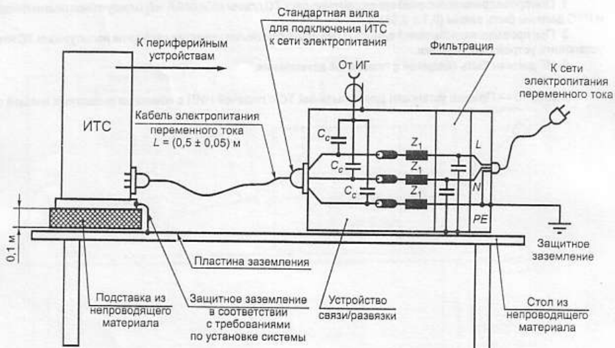
Рисунок 11 — Пример установки для испытаний стационарного напольного ТС на месте эксплуатации с подачей НИП на порты электропитания переменного и постоянного тока и порт защитного заземления
