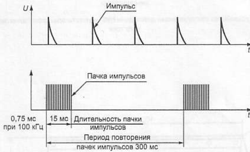
Рисунок 2 — Пачки НИП
