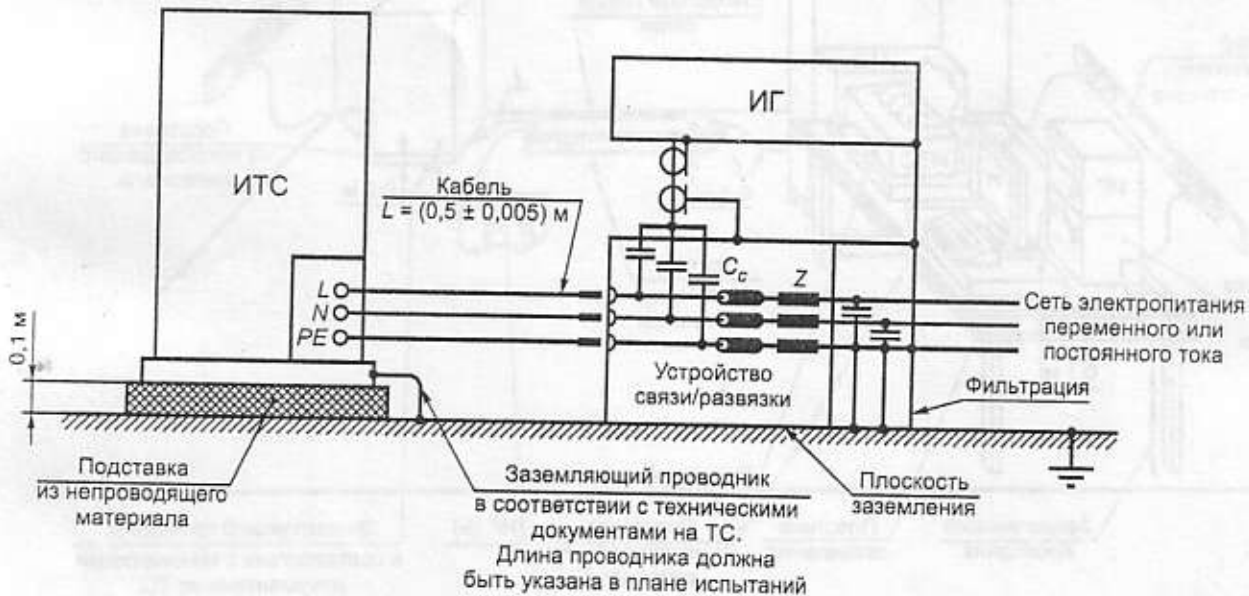
Рисунок 8 — Пример установки для испытания оборудования в стойке
