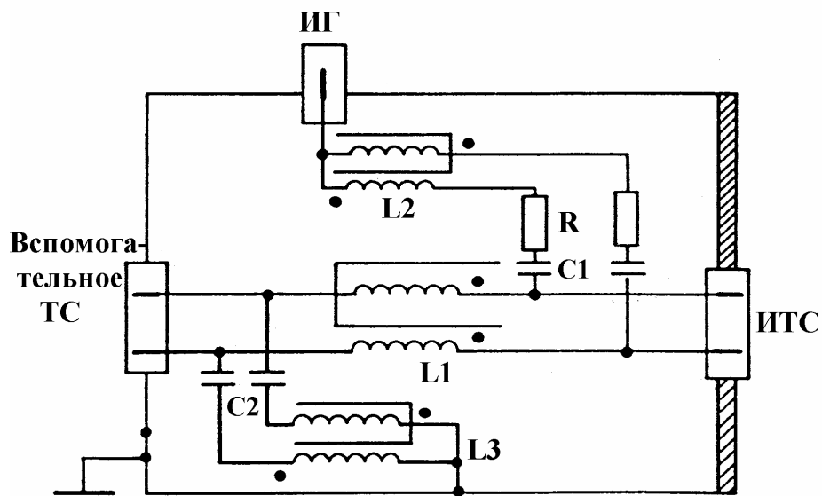
Рисунок Г.3 - Упрощенная схема устройства связи / развязки типа УСР-НС2, применяемого при вводе помехи в неэкранированные несимметричные линии (см. 6.2.2.3)
