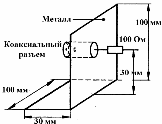
Рисунок 6 б - Схема установки для проверки полного сопротивления общего вида устройств связи / развязки
